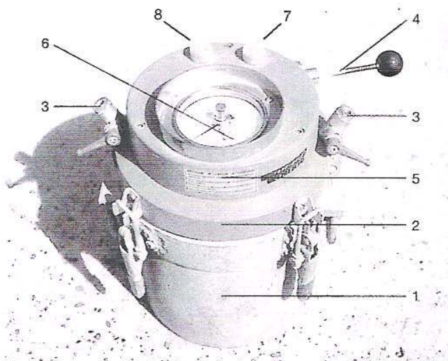
Bild 5: Druckausgleichsverfahren (LP-Topf)
