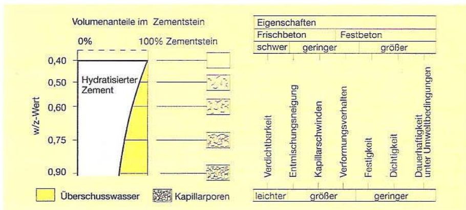
Bild 1: Frisch- und Festbetoneigenschaften in Abhängigkeit vom Wasserzementwert
